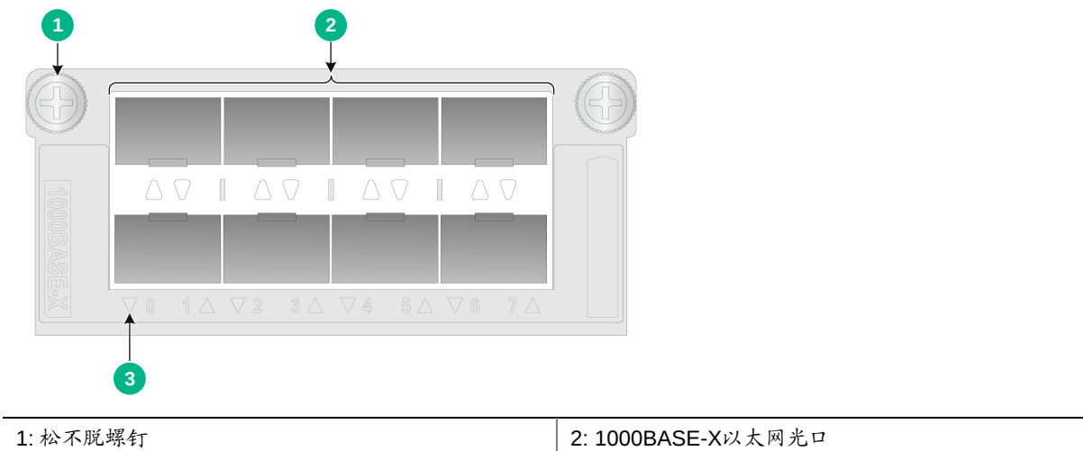
图A-6 NS-NIM-GP8B-Z 接口模块正视图
