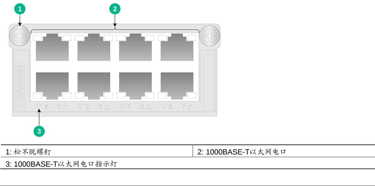
图A-5 NS-NIM-GT8B-Z 接口模块正视图
