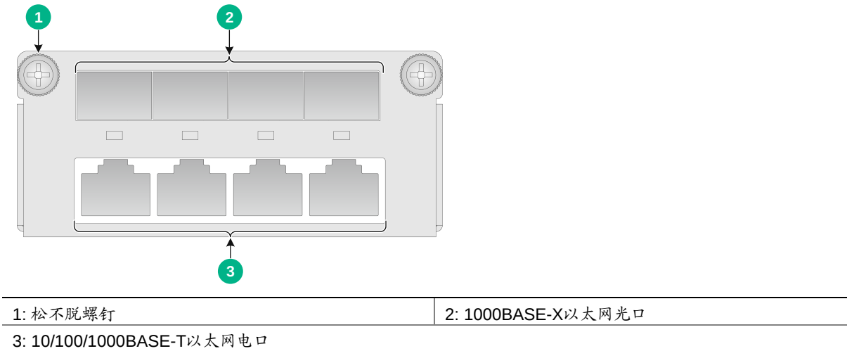
图A-3 NS-NIM-GT4GP4A-Z 接口模块正视图
