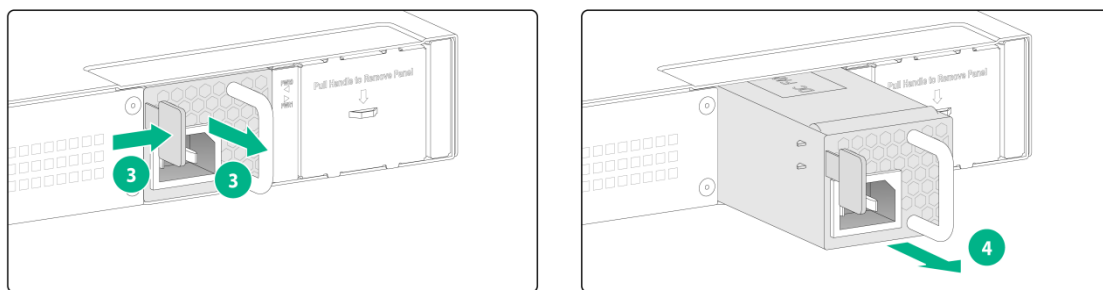
图4-2 拆卸电源模块
