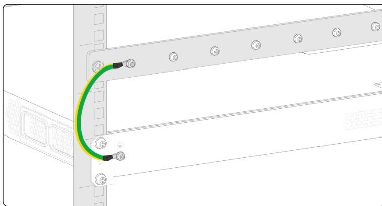
图2-9 连接到机柜接地
